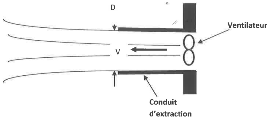
Figure 2 : Extracteur d'air vu en coupe
